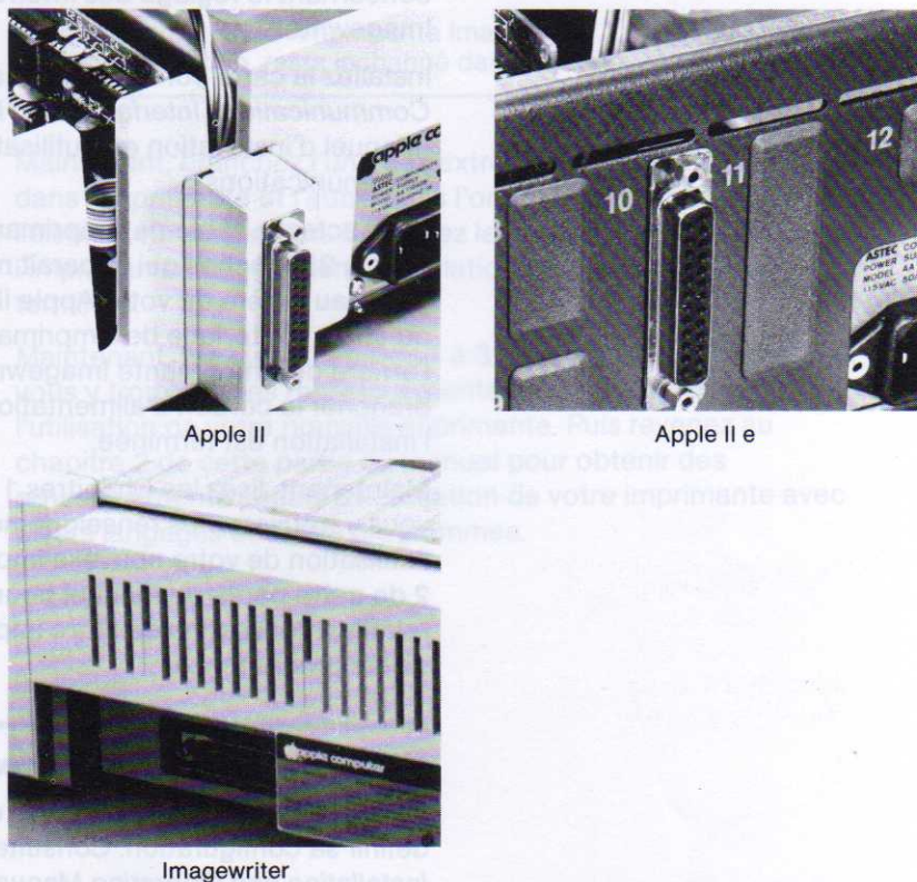
Figure 1-2. Connecteurs d'interface série de l'Apple II/IIe
